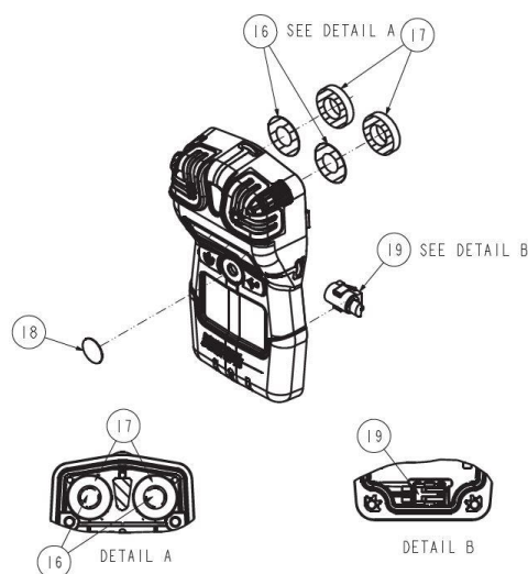
Abbildung 6.2. Demontiertes Gehäuseoberteil des TX1
