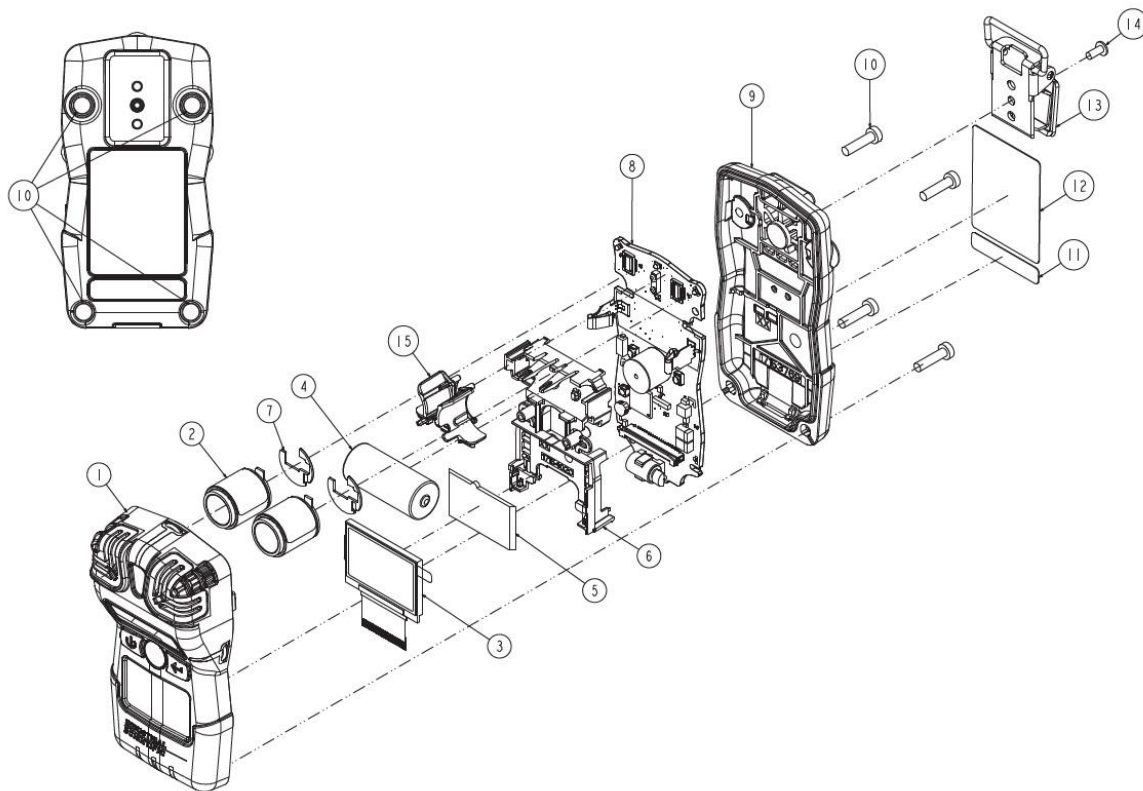
Abbildung 6.1. Demontiertes Tango TX1
